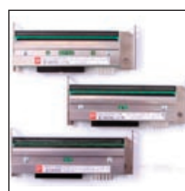
Individuell konfigurierbarer Druckkopf (203dpi / 305dpi / 609dpi). Justierbar auf Knopfdruck
